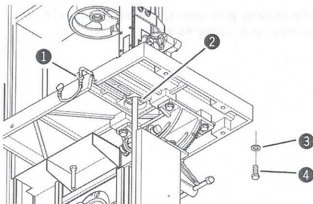
Fig. 6-2: Work table
